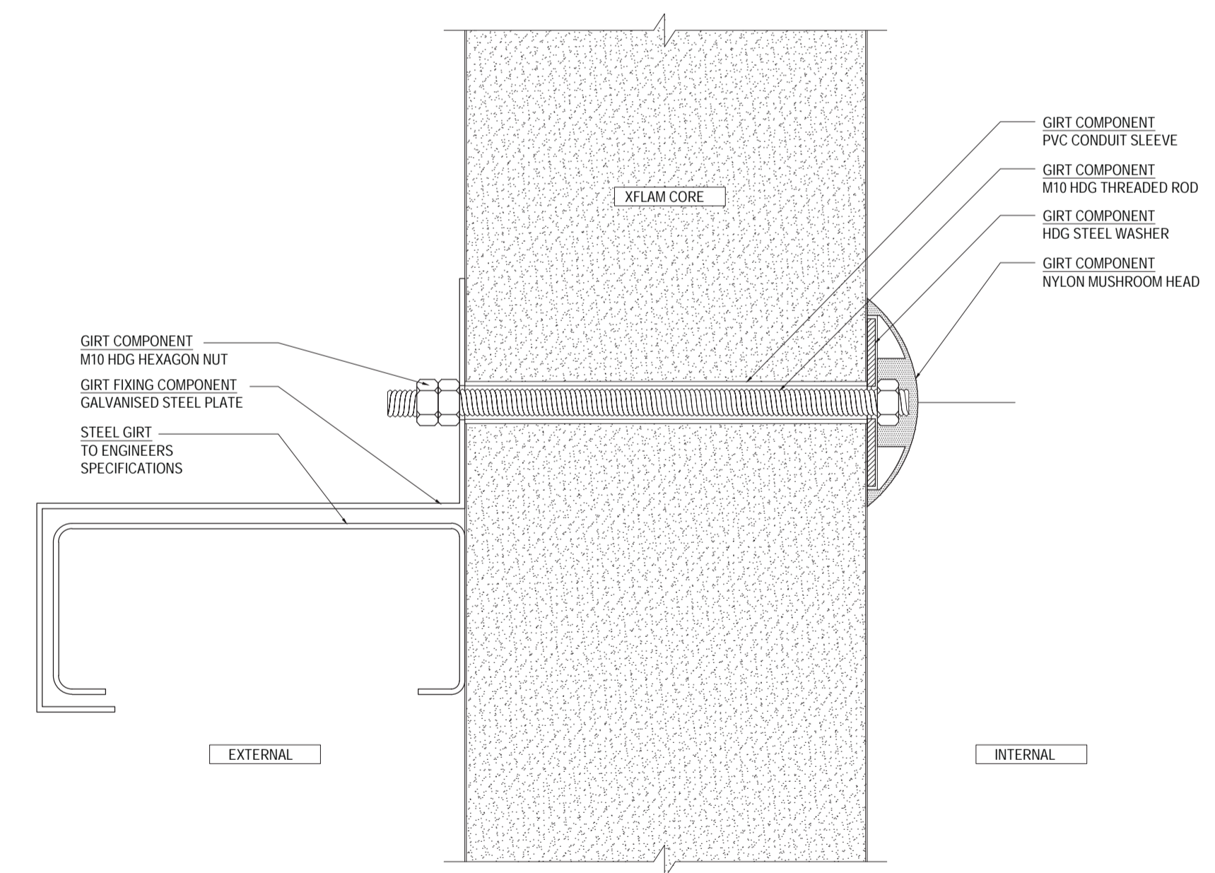
IWC-XGA-ML-03 SCALE 1:2
