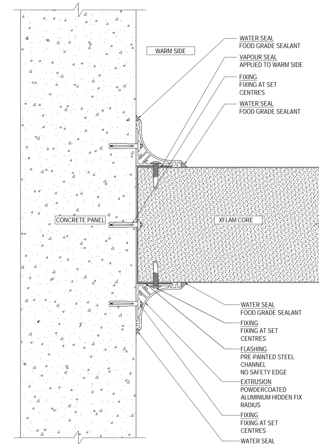
IWC-XWW-IN-AT-04 SCALE 1:2
