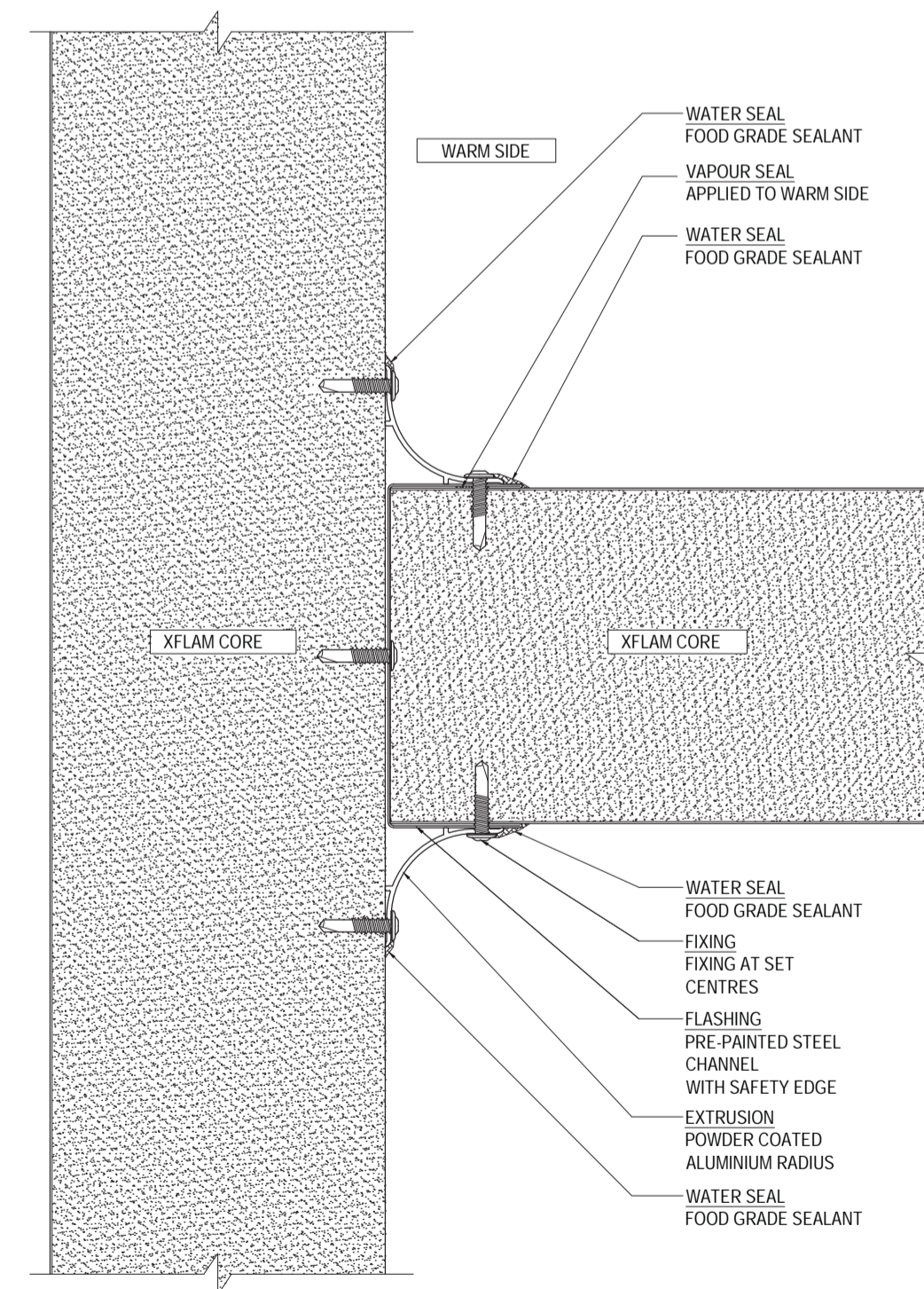
IWC-XWW-IN-AT-07 SCALE 1:2
