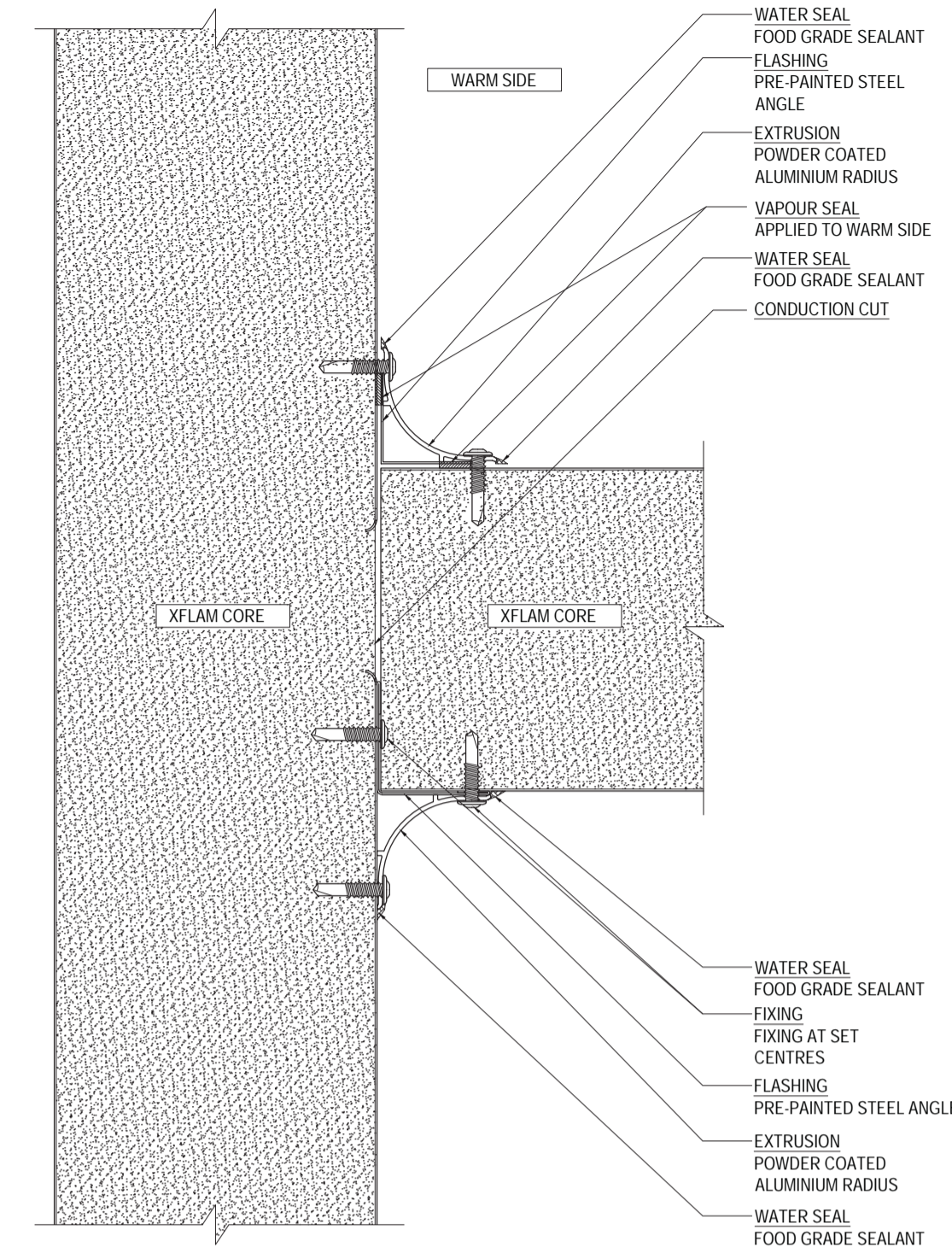
IWC-XWW-IN-ML-07 SCALE 1:2
