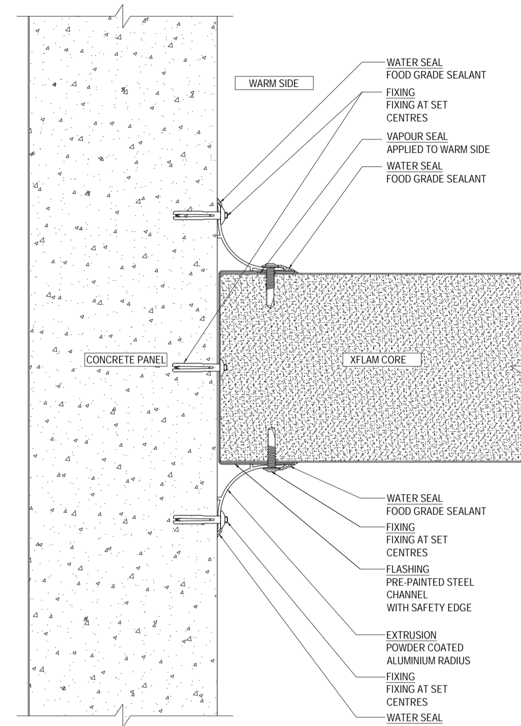
IWC-XWW-IN-AT-03 SCALE 1:2
