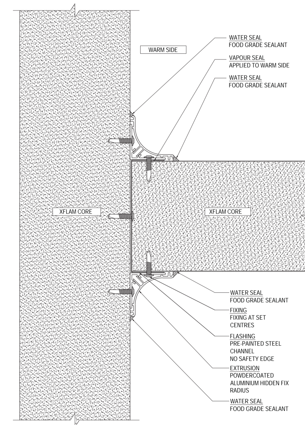
IWC-XWW-IN-AT-08 SCALE 1:2
