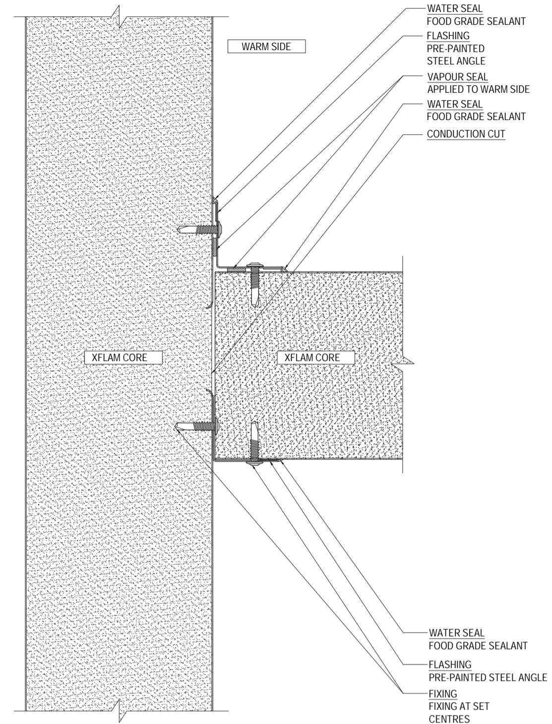
IWC-XWW-IN-ML-05 SCALE 1:2
