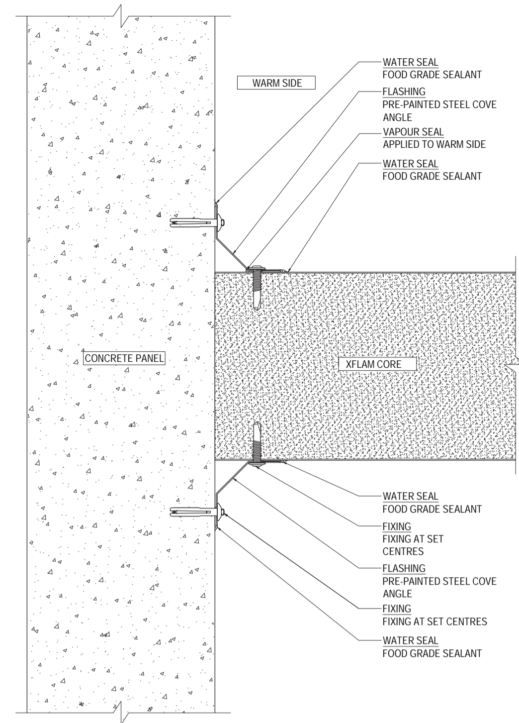
IWC-XWW-IN-AT-02 SCALE 1:2
