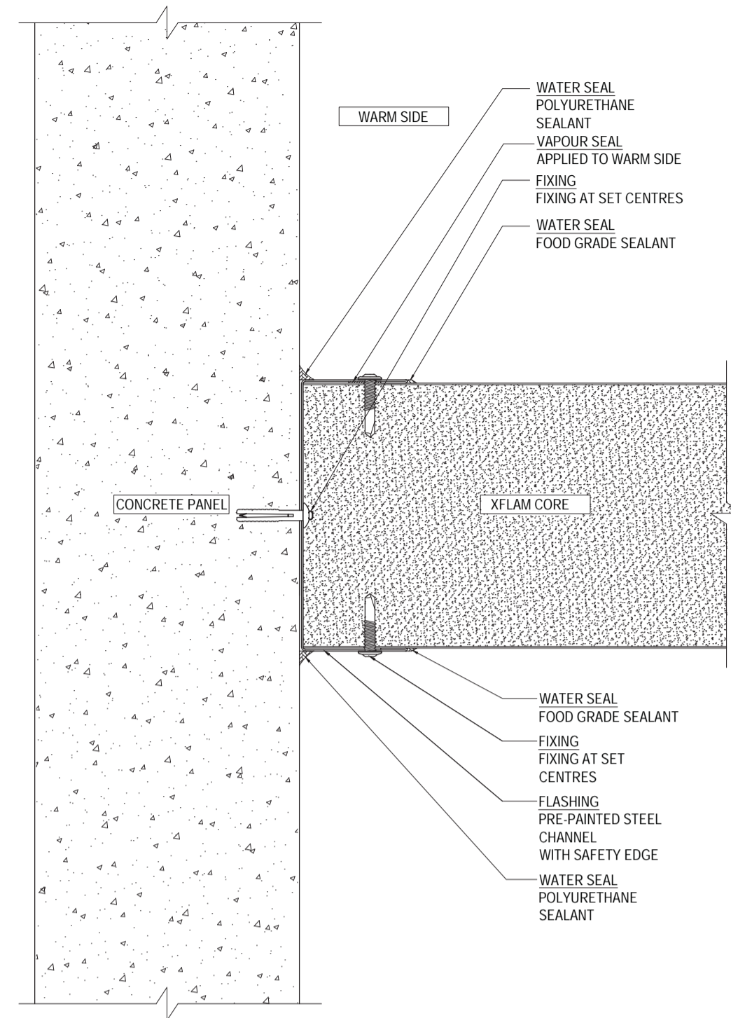
IWC-XWW-IN-AT-01 SCALE 1:2
