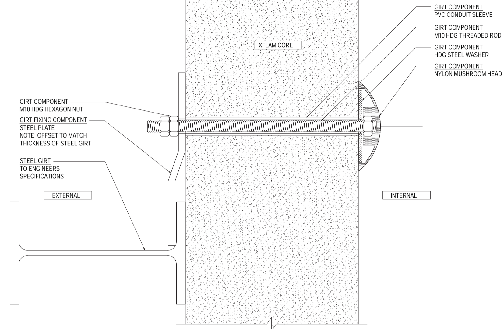
IWC-XGA-ML-02 SCALE 1:2
