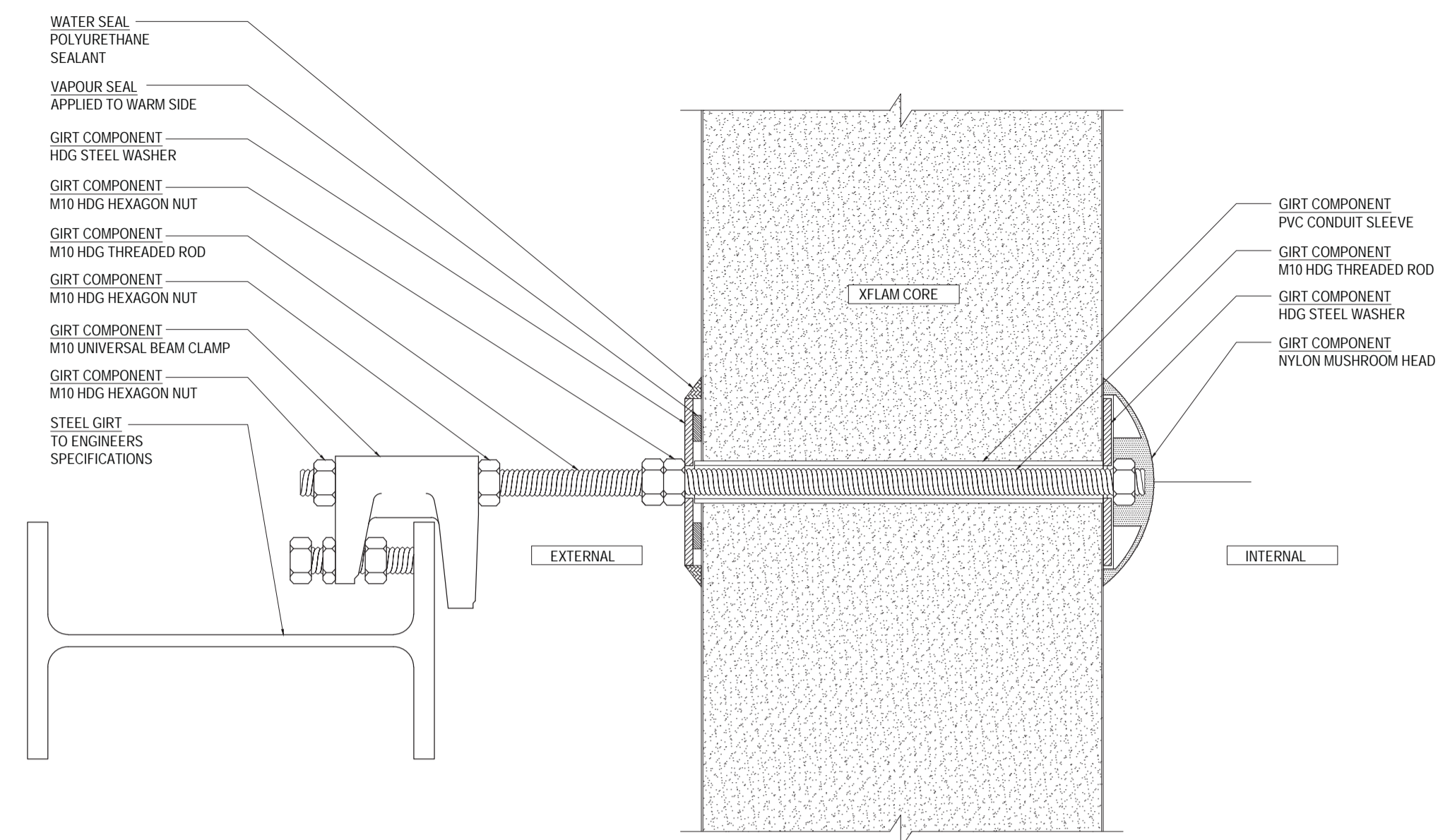
IWC-XGA-ML-01 SCALE 1:2
