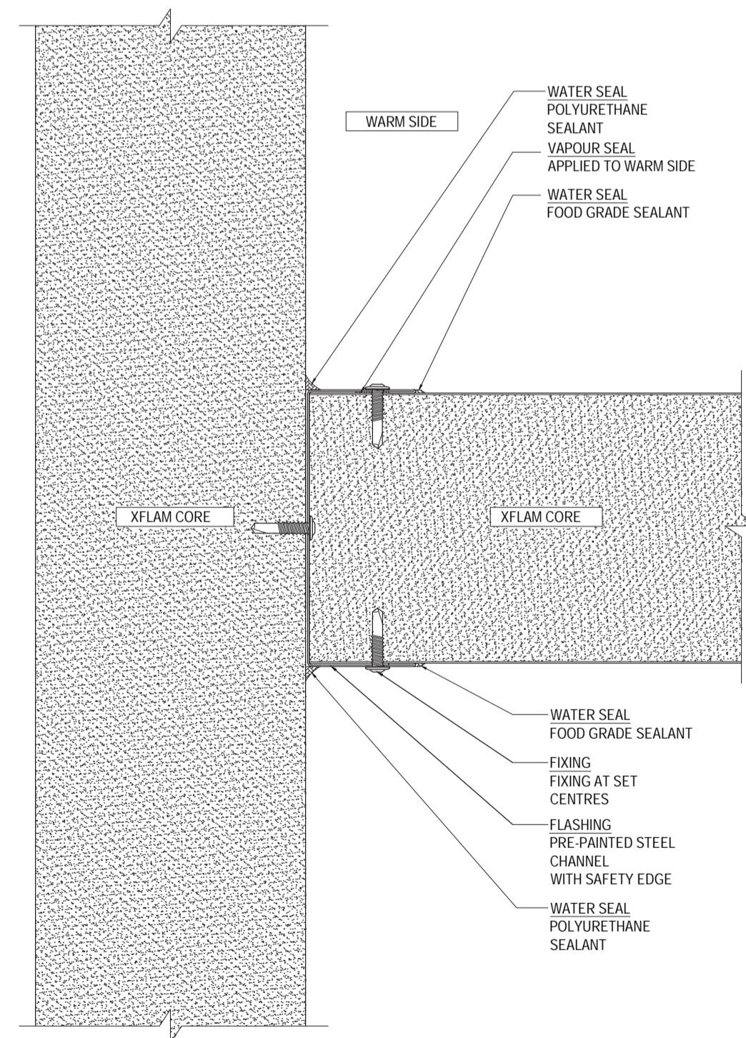
IWC-XWW-IN-AT-05 SCALE 1:2
