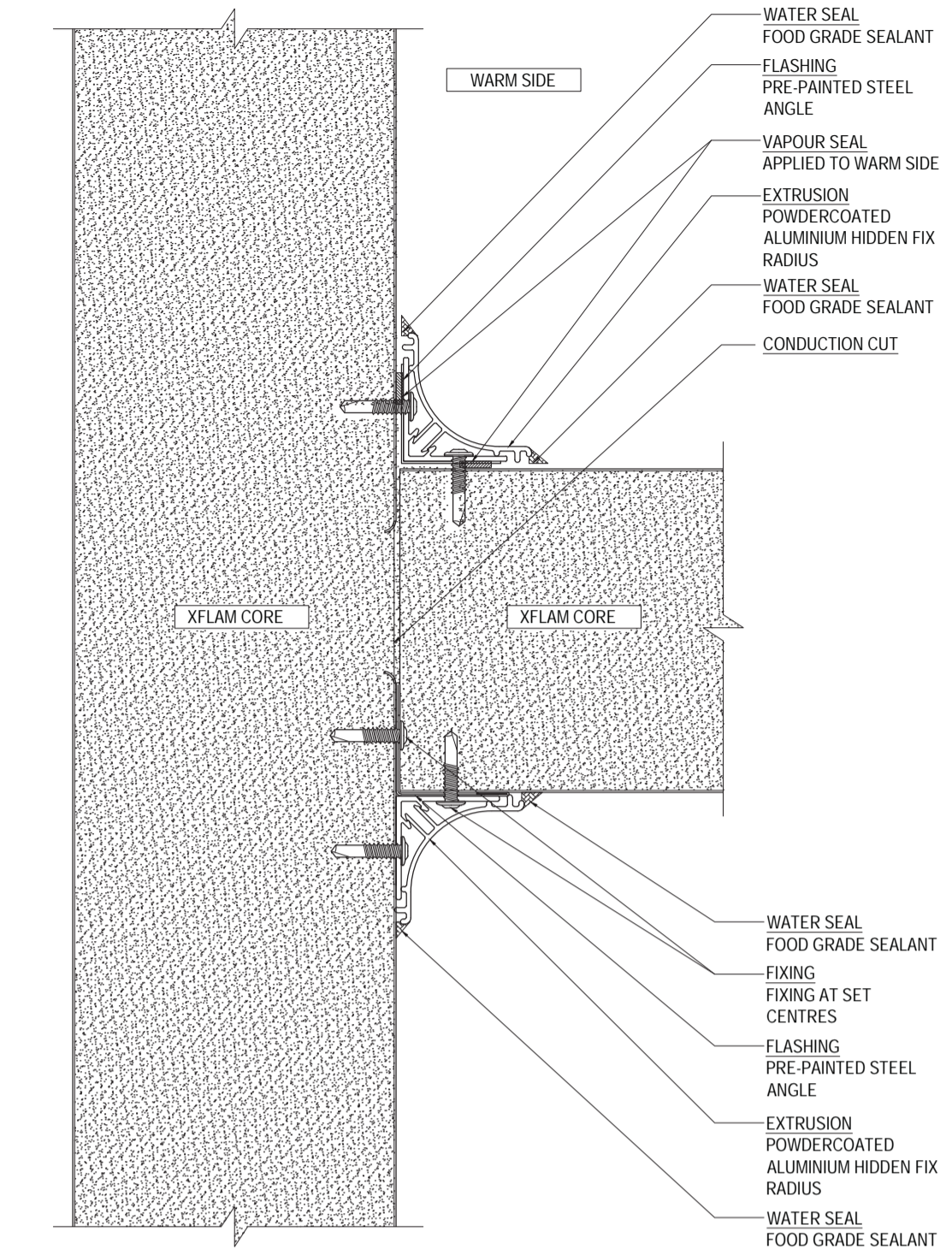
IWC-XWW-IN-ML-08 SCALE 1:2
