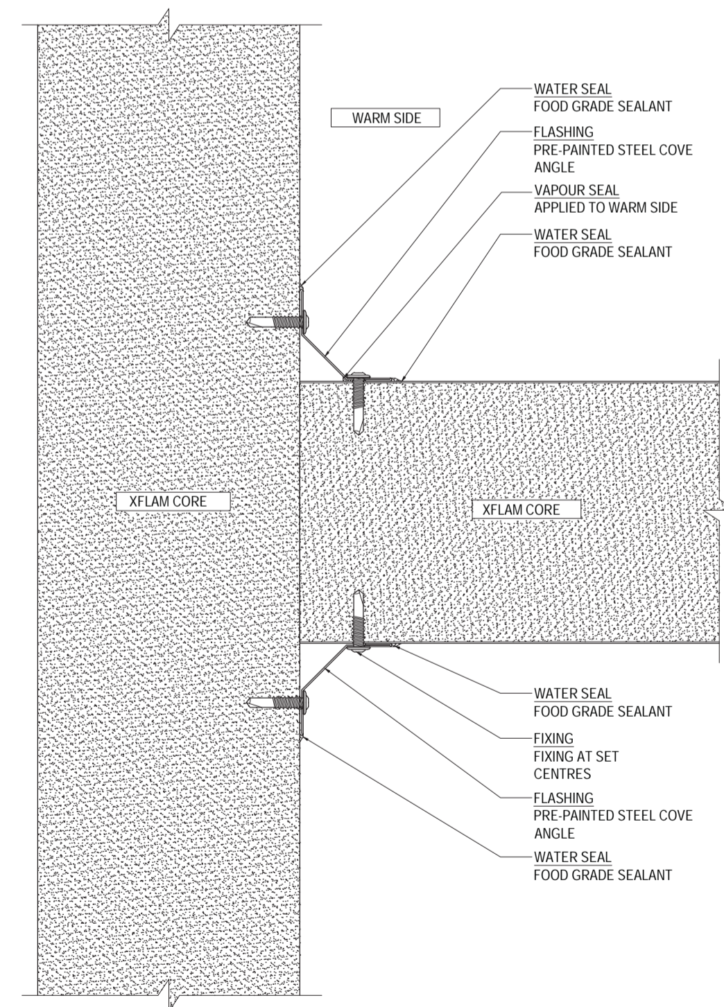
IWC-XWW-IN-AT-06 SCALE 1:2
