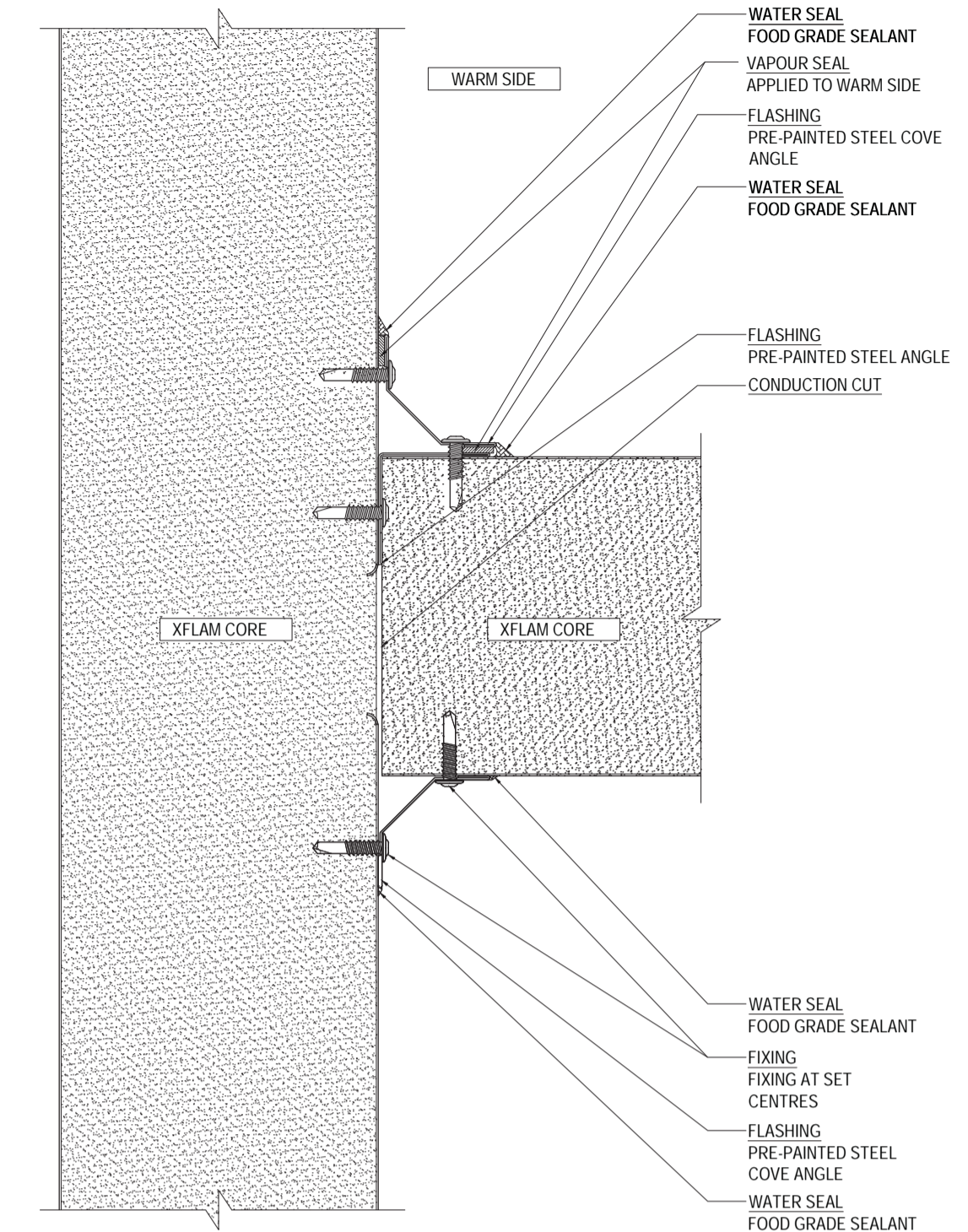
IWC-XWW-IN-ML-06 SCALE 1:2
